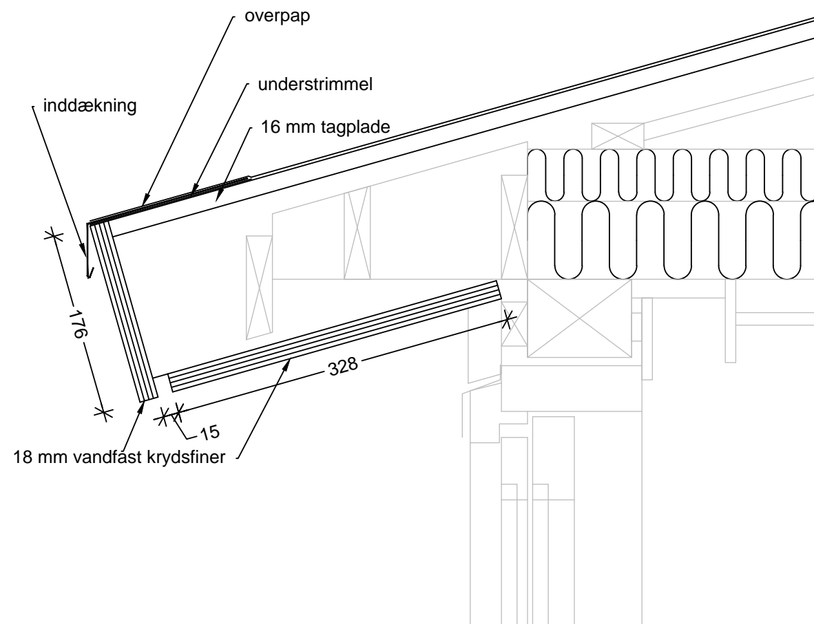
Principalsnit til etape 1, rød bygning
