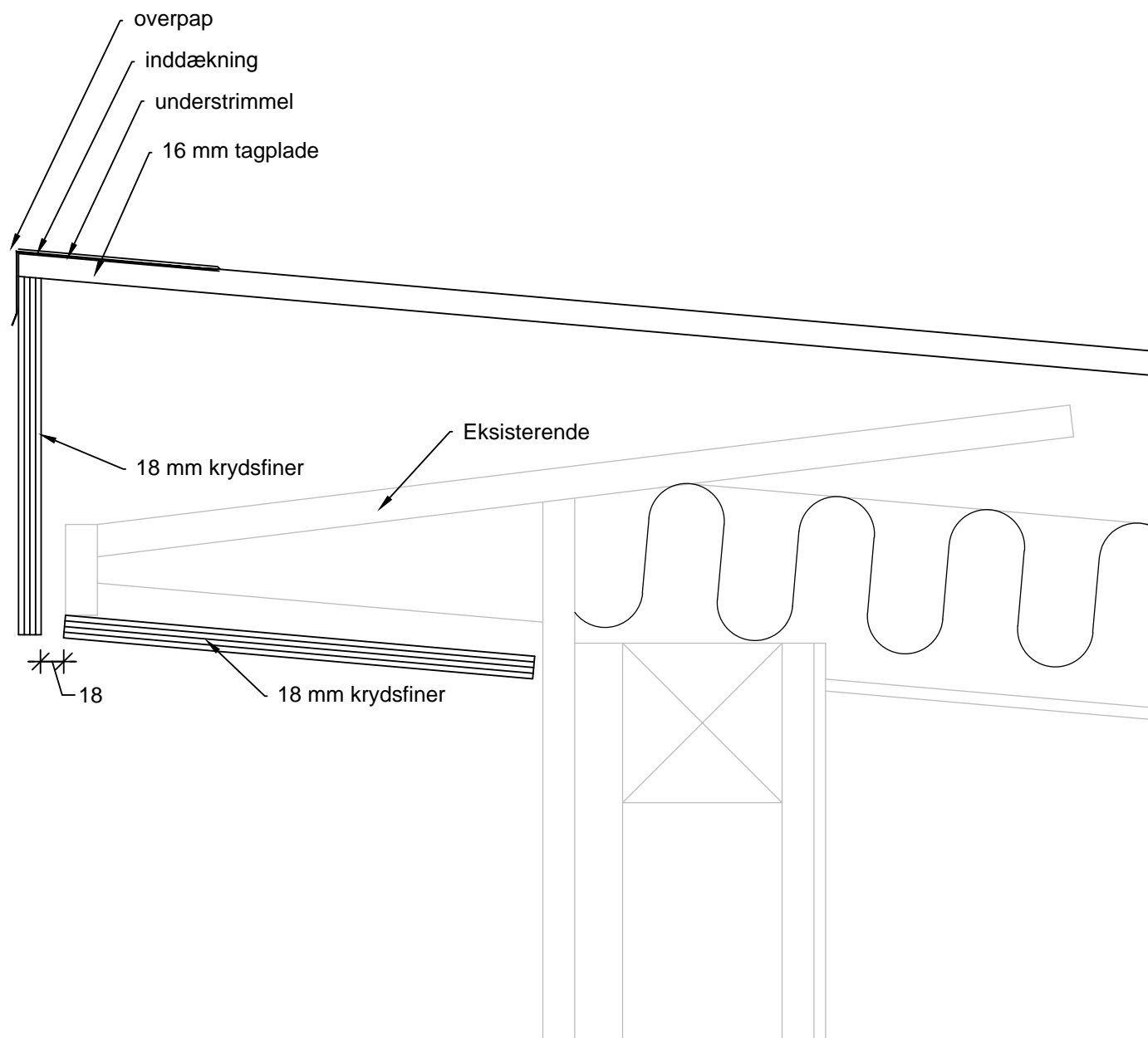
Principalsnit til etape 2, grøn bygning og etape 3, mellembygning
