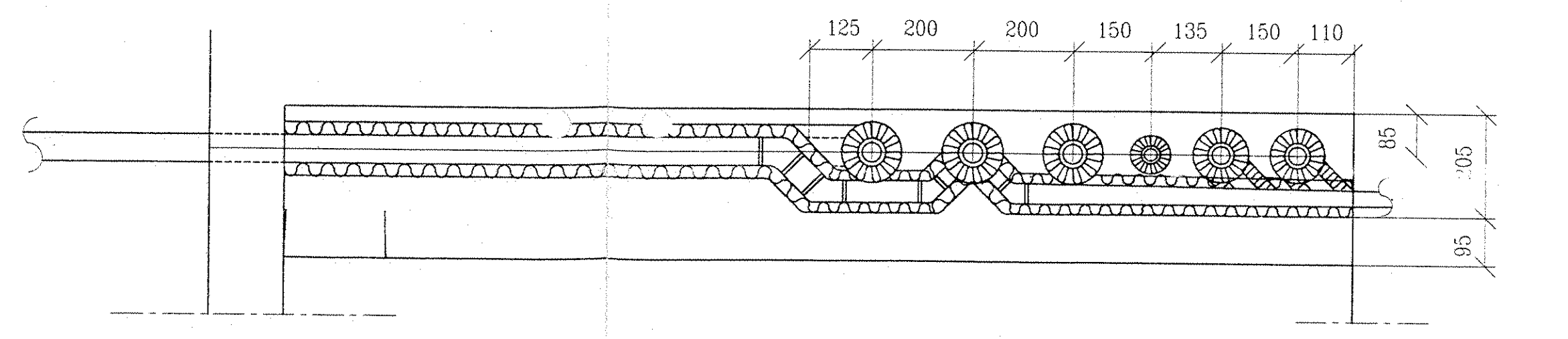
PRINCIPSNI I GANG OVER NEDHÆNGT LOFT, 1:10
