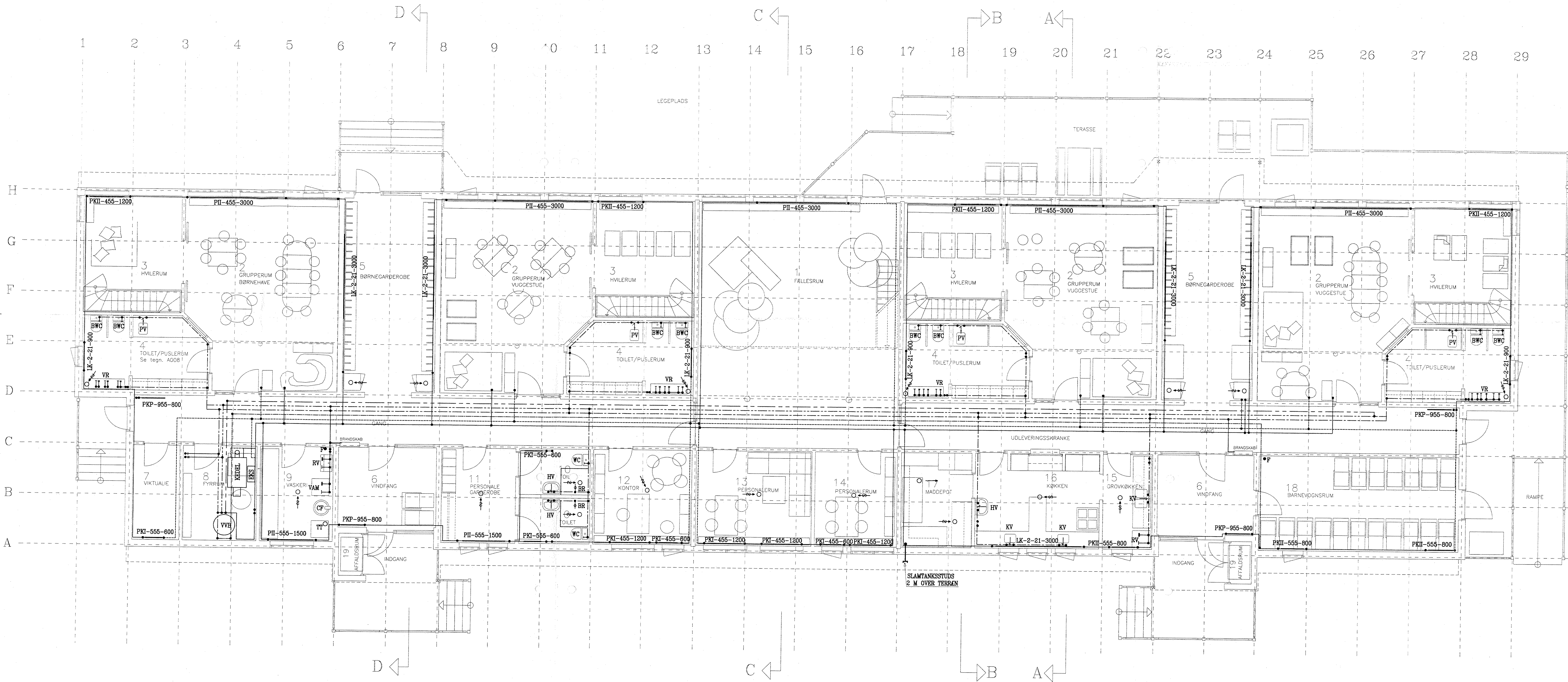
STUEPLAN, 1:50
